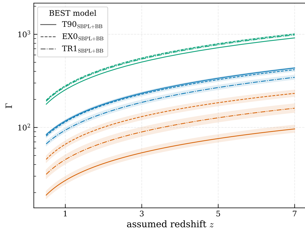
GRB231129C
