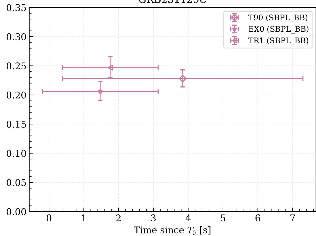
GRB231129C
