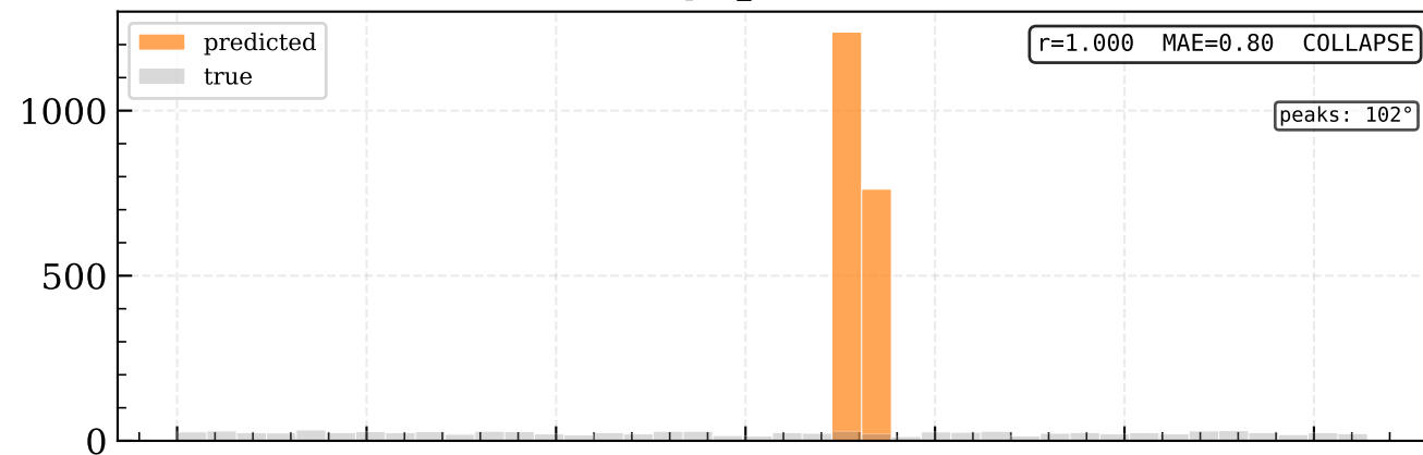
poc_b (PoC)
