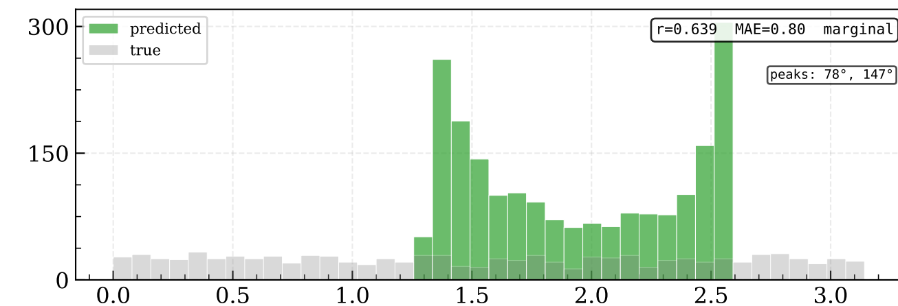
tcn
