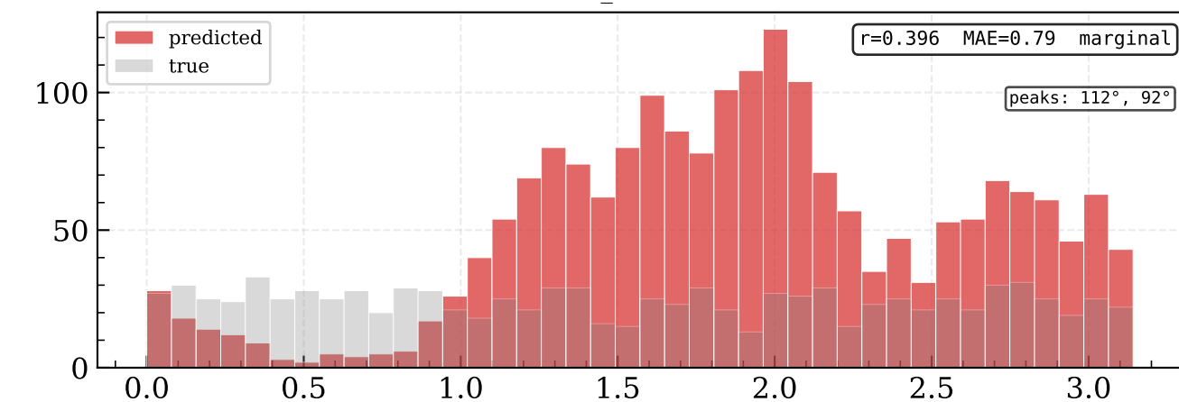
cnn_attention
