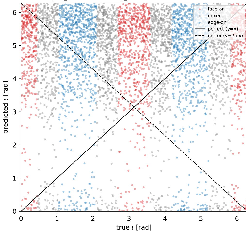
tcn (ang_MAE=1.5400, null=1.5708)
