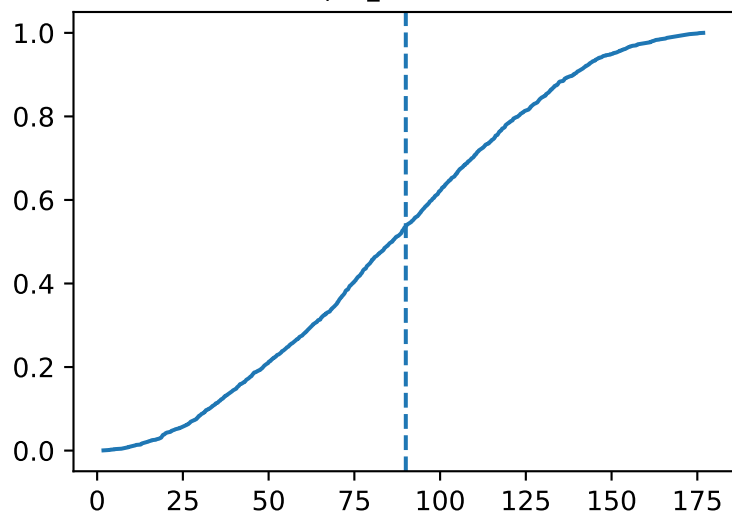
poc_b — CDF
