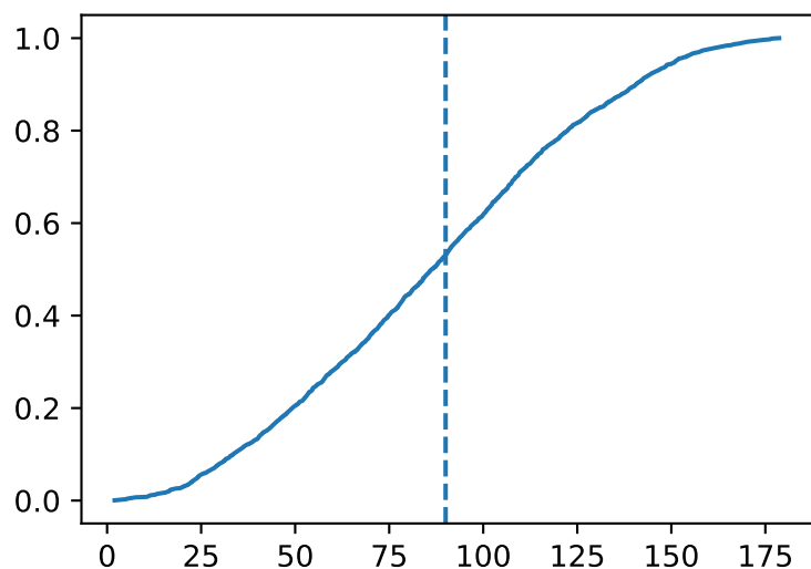
cnn_attention — CDF
