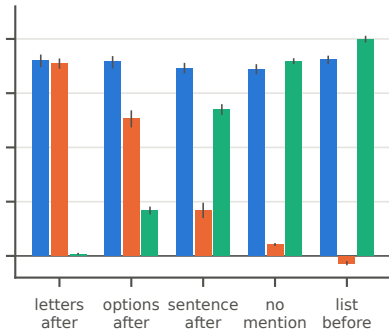
(b) Qwen2.5-72B
