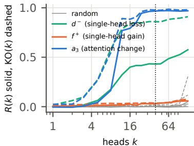
Qwen2.5-7B, options-after
