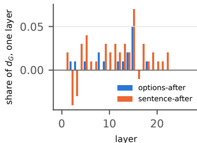
Qwen2.5-7B, layer profile
