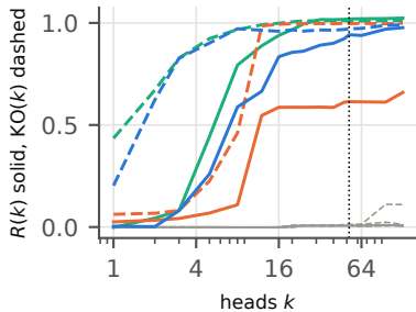
Mistral-7B, options-after
