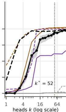
Mistral-7B
