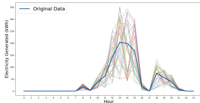
Figure 7: 시나리오별 개별 DER의 발전량
