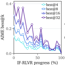
(a) AIME searchability
