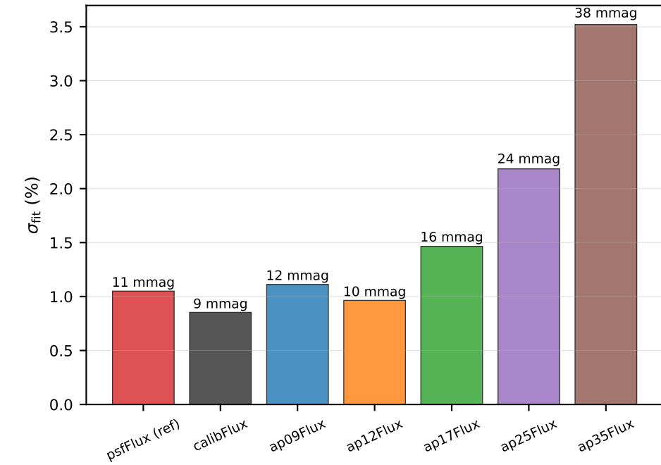
y band
