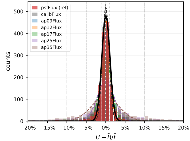
y band
