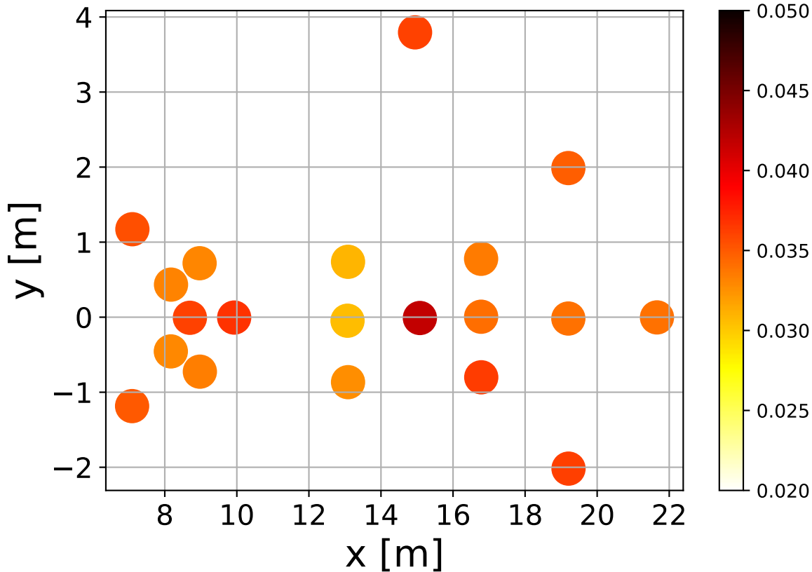
Model1.33 s
