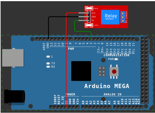
Gambar 30: Rangkaian simulasi modul relai daya satu saluran terisolasi optik pada platform Wokwi.
