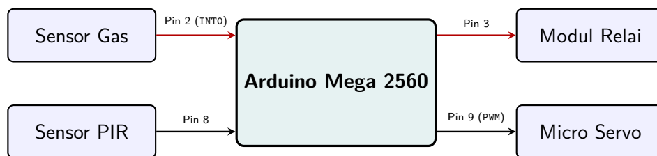
Gambar 40: Diagram blok antarmuka periferi dan aktuator sistem.
