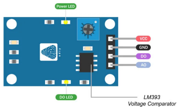
Gambar 18: Pemetaan pin dan antarmuka modul sensor MQ.
