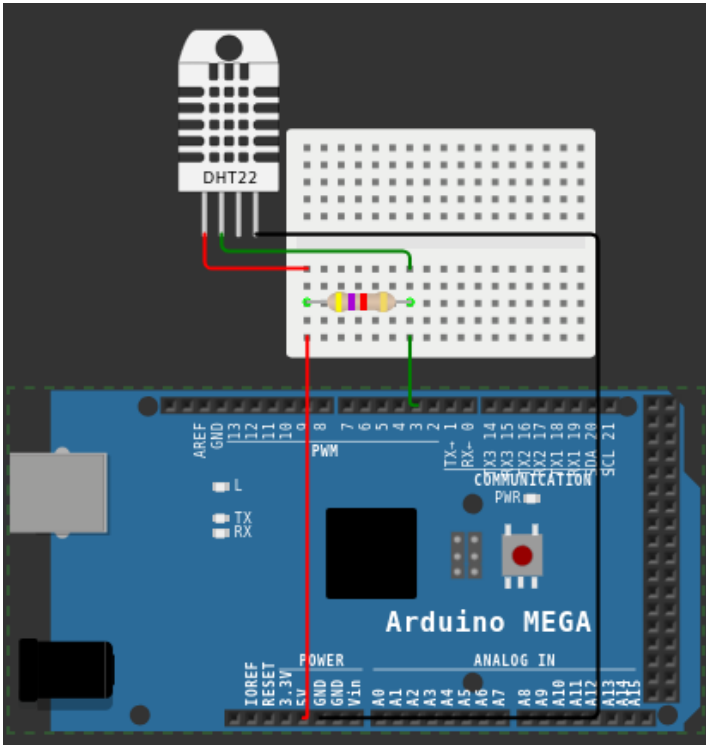
Gambar 13: Rangkaian sensor DHT22/AM2302 dengan mikrokontroler ATmega2560 pada simulasi Wokwi.
