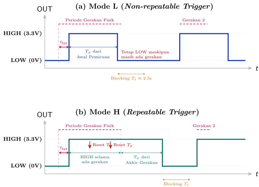
Gambar 23: Perbandingan mekanisme perhitungan waktu tunda T_x dan latensi deteksi t_{lat} pada Mode L ( Non-repeatable ) dan Mode H ( Repeatable ).
