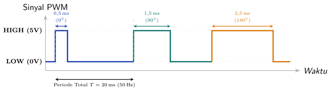
Gambar 33: Diagram pewaktu sinyal kontrol PWM dan durasi pulsa pemicu sudut posisi servo SG90.
