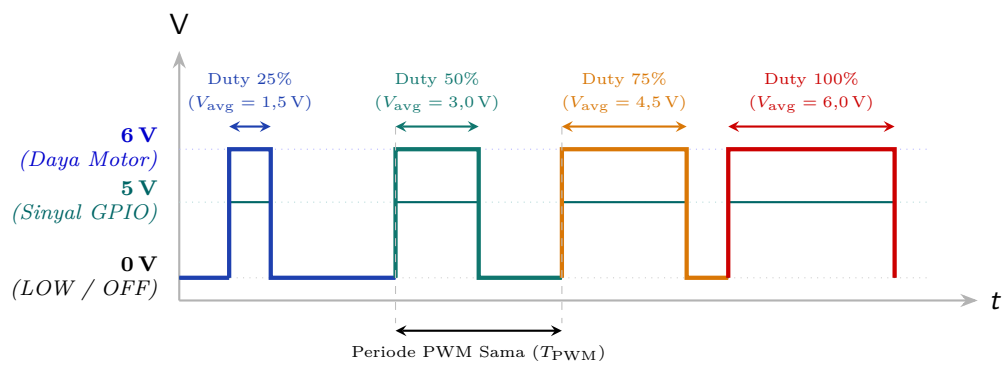
Gambar 38: Diagram pewaktu sinyal kontrol PWM dari GPIO (5 V) dan keluaran sakelar daya driver (6 V) pada mikro DC motor.
