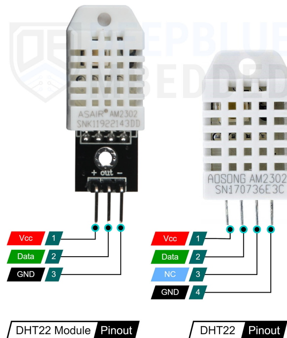
Gambar 12: Pemetaan pin dan antarmuka komponen AM2302/DHT22.
