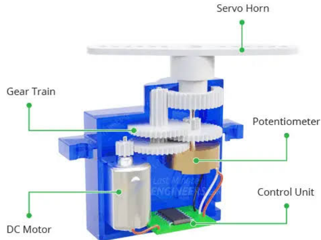
Gambar 32: Struktur sirkuit kendali tertutup internal motor servo SG90.
