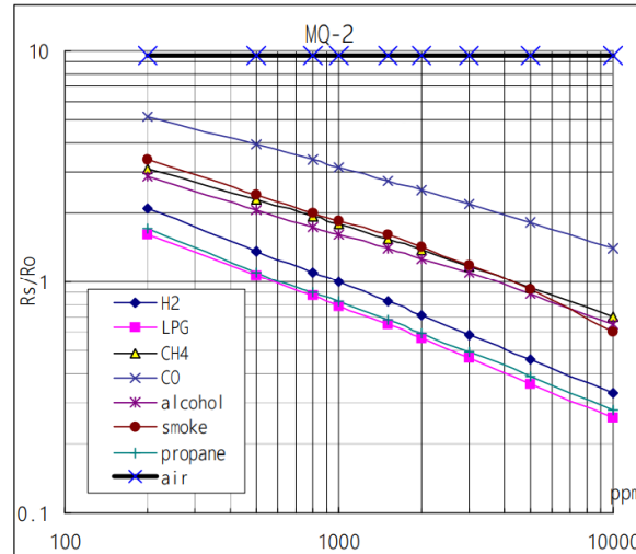
Gambar 15: Kurva karakteristik sensitivitas sensor MQ-2.
