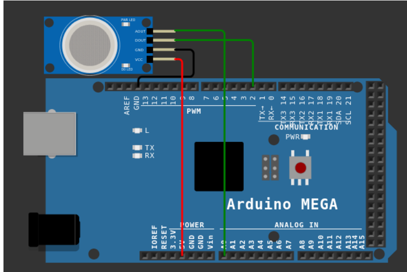
Gambar 19: Rangkaian demonstrasi sensor MQ-2 / MQ-135 dengan Arduino Mega 2560 pada simulasi wokwi.
