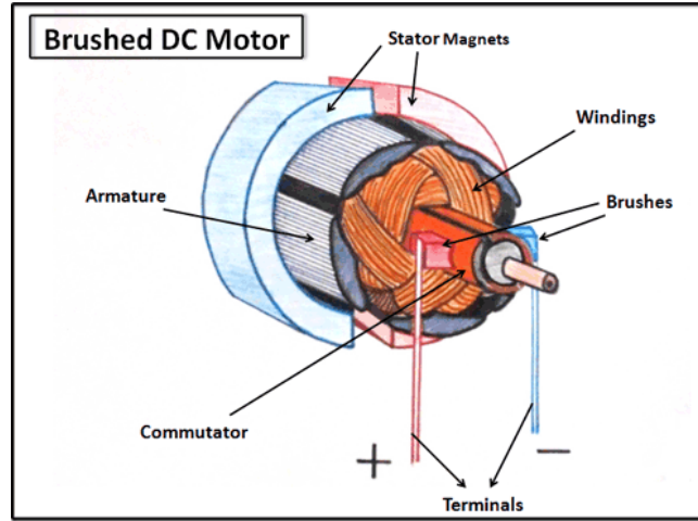
Gambar 37: Struktur internal motor DC bersikat.
