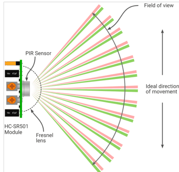
Gambar 22: Sudut deteksi dan arah pergerakan optimal sensor PIR HC-SR501.
