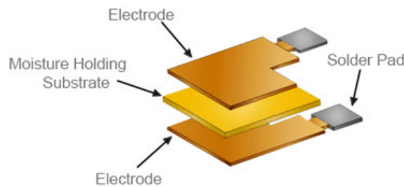
Gambar 9: Komponen internal elemen sensoris kelembapan pada DHT22.
