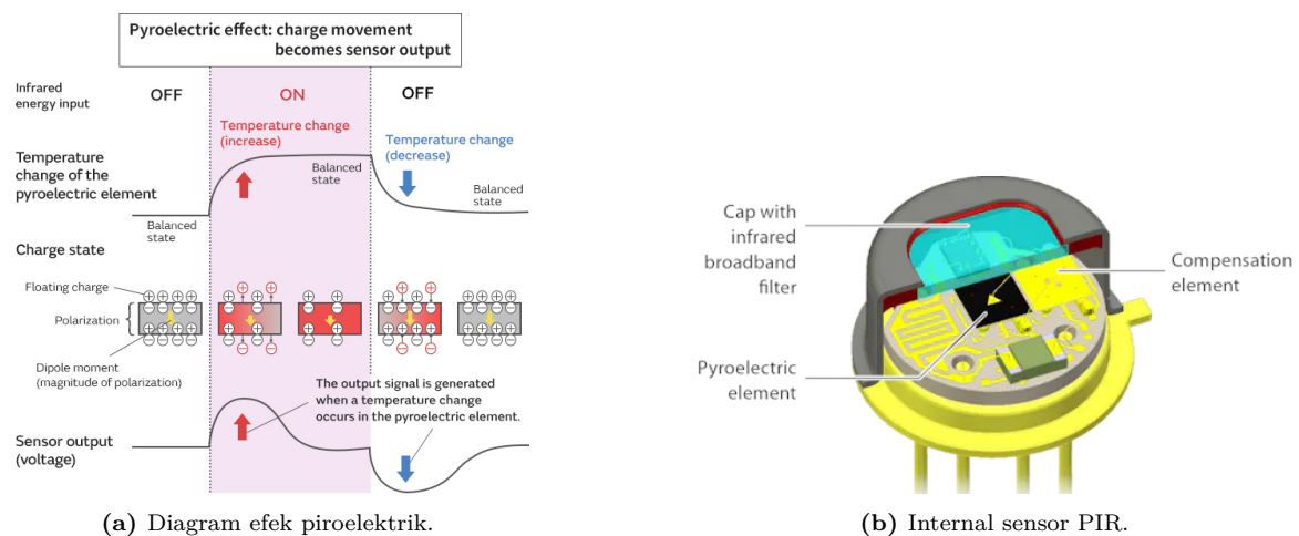
Gambar 21: Prinsip kerja dan diagram internal elemen sensoris pada HC-SR501.
