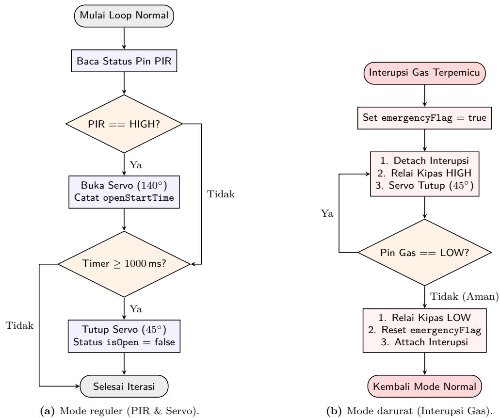
Gambar 41: Diagram alur logika eksekusi sistem: (a) Mode operasional harian berbasis PIR dan (b) Mode penanganan kebocoran gas berbasis interupsi.
