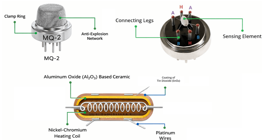
Gambar 16: Komponen internal dan elemen sensoris modul sensor MQ.
