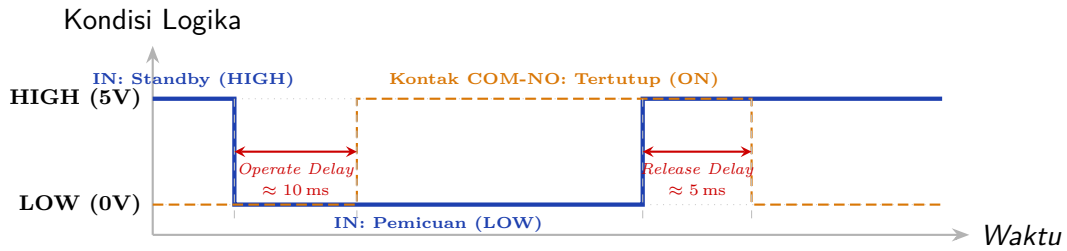
Gambar 28: Diagram pewaktu sinyal kontrol pemicuan Active-LOW dan respons tanggapan kontak mekanis relai JQC-3FF-S-Z.
