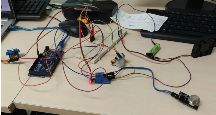
Gambar 42: Rangkaian Sistem Deteksi Gas & Penanganan Darurat Otomatis.
