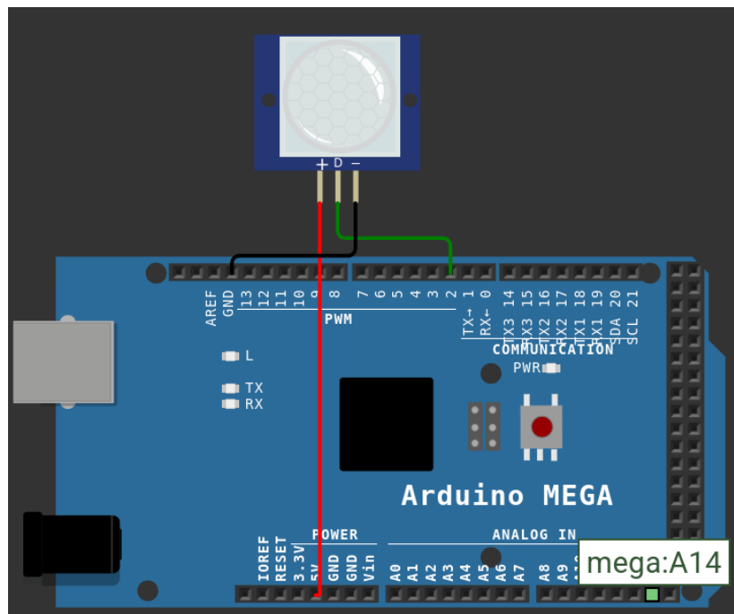
Gambar 25: Rangkaian antarmuka modul HC-SR501 dengan Arduino Mega 2560 pada simulasi Wokwi.
