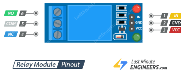
Gambar 29: Pemetaan pin dan antarmuka modul JQC-3FF-S-R relai daya.
