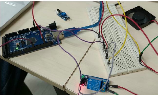
Gambar 39: Contoh rangkaian pengontrolan kipas DC menggunakan modul relai.
