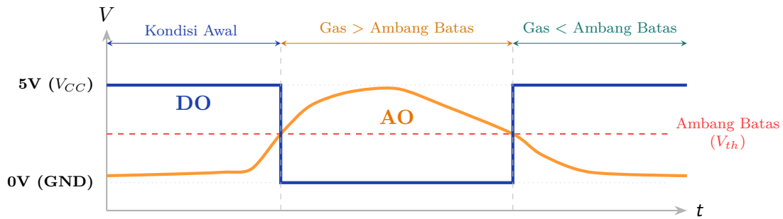
Gambar 17: Karakteristik perbandingan output sinyal analog (AO) dan digital (DO) pada modul sensor MQ.
