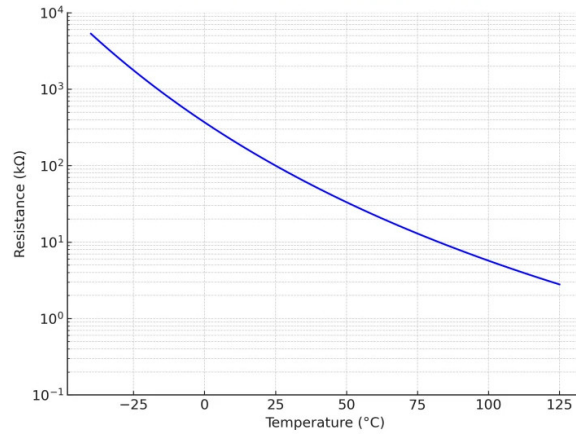
Gambar 8: Kurva karakteristik hubungan suhu terhadap resistansi pada NTC Thermistor.
