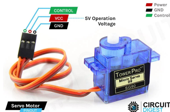
Gambar 34: Pemetaan pin dan antarmuka modul mikro servo SG90.
