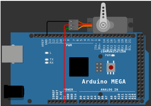
Gambar 35: Rangkaian simulasi pengujian servo pada platform Wokwi.
