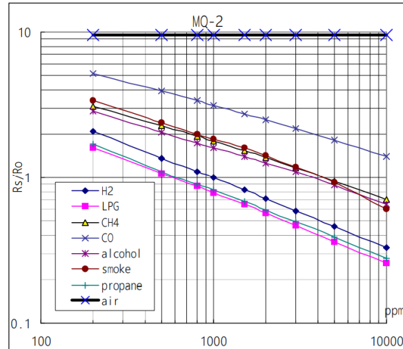
Gambar 15: Kurva karakteristik sensitivitas sensor MQ-2.
