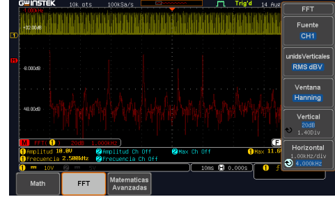
Figura 5. Armónicos presentes en la señal reconstruida con una frecuencia de muestreo de 2.5 kHz.
