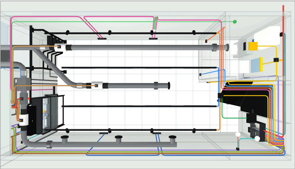
Top view (walls transparent)
