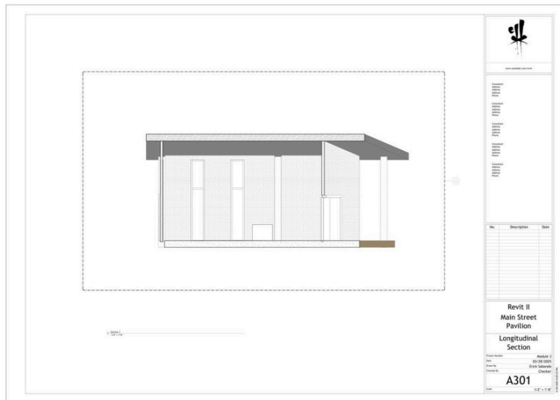
LONGITUDINAL SECTION - A301
