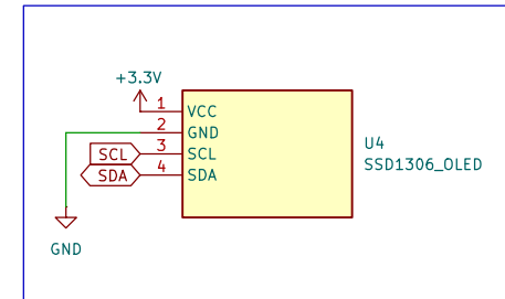
Display
