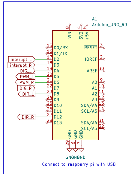
Arduino_Uno_Core
