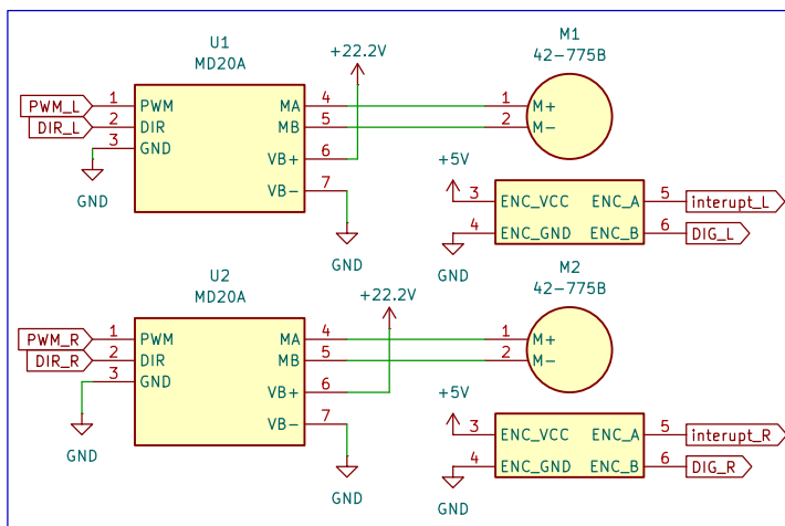
Motor
