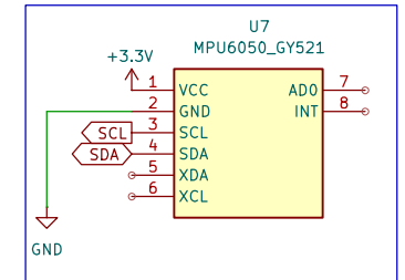
IMU_Interface
