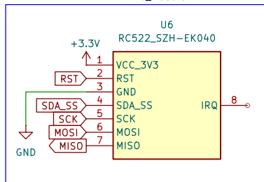
NFC_Module
