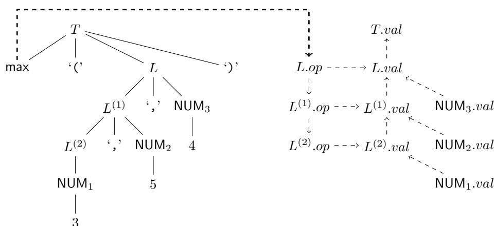
図 6.9: 属性の評価
