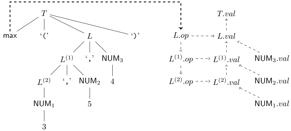
図 6.8: 属性の評価
