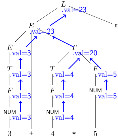
図 6.7: 解析木と属性評価
