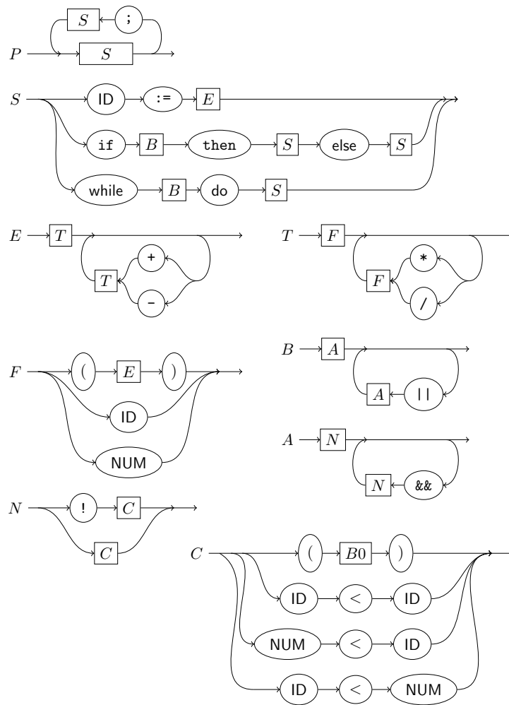
図 6.6: P の構文図式
