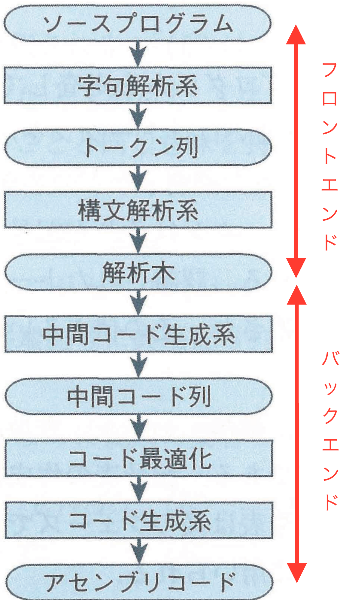
図 2.1 コンパイラの構造
