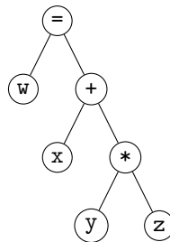
図 6.2: 抽象構文木の例
