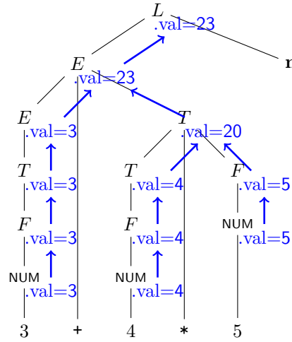
図 6.9: 解析木と属性評価
