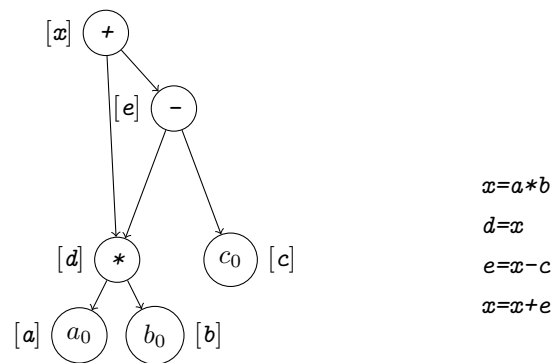
(d) 不要コード消去の適用
