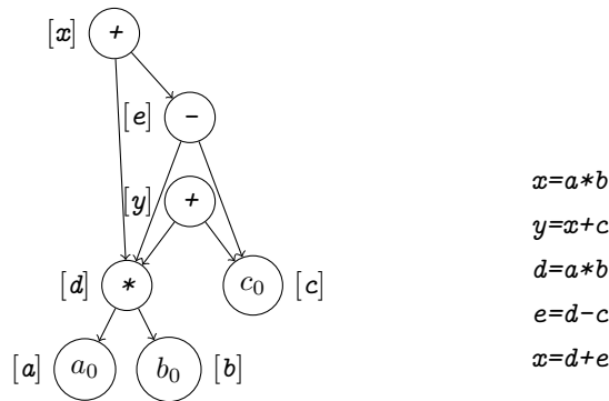
(b) 5 行目までで生成される DAG
