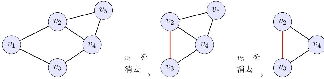
図 1.7: グラフ頂点の消去操作
