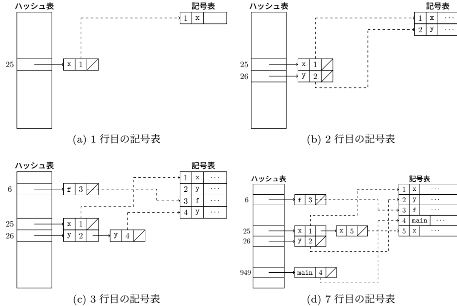
図 5.3: コンパイルの過程における記号表の構成
