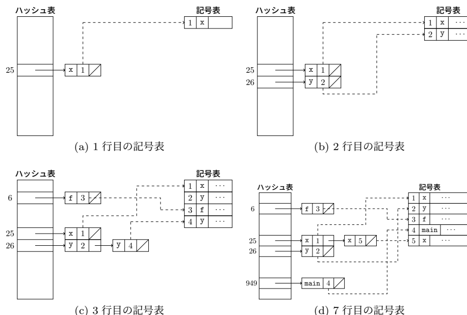
図 5.2: コンパイルの過程における記号表の構成
