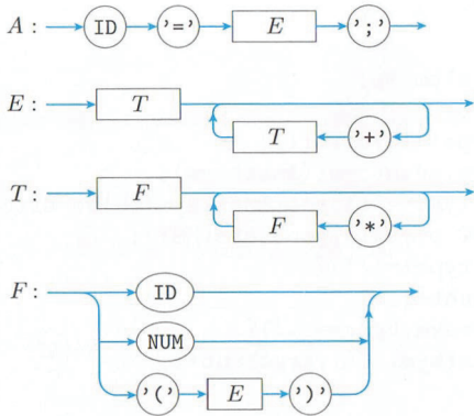
図 5.13 代入文の構文図式
