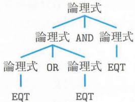
図 4.1 2通りの解析木
