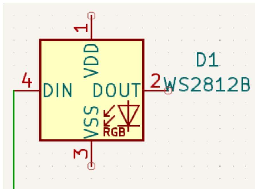
Рисунок 11 – Модуль WS2812b из библиотеки LED
