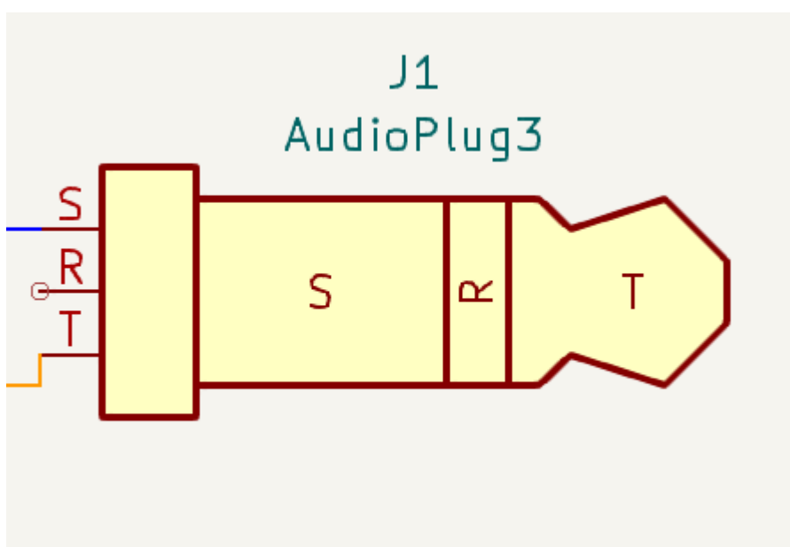
Рисунок 12 – Модуль AudioPlug3 из библиотеки Connector_Audio
