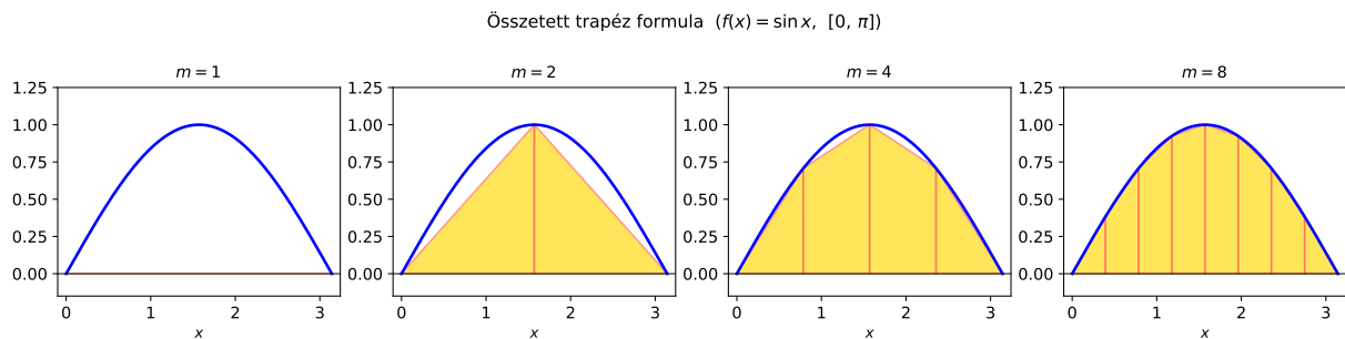
2. ábra. Az összetett trapéz formula m = 1, 2, 4, 8 résszel (f(x) = \sin x, [0, \pi]) . Az arany színű terület a közelítő, a kék görbe az egzakt függvény.
