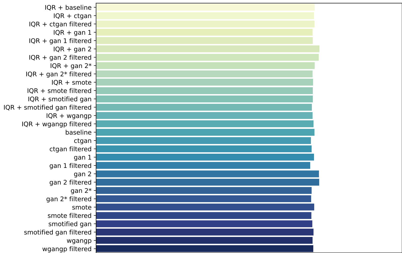
NSL-KDD
