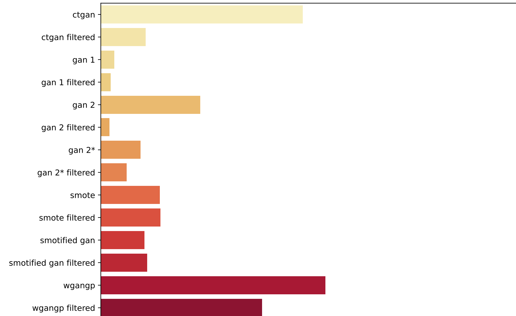
IQR Madelon
