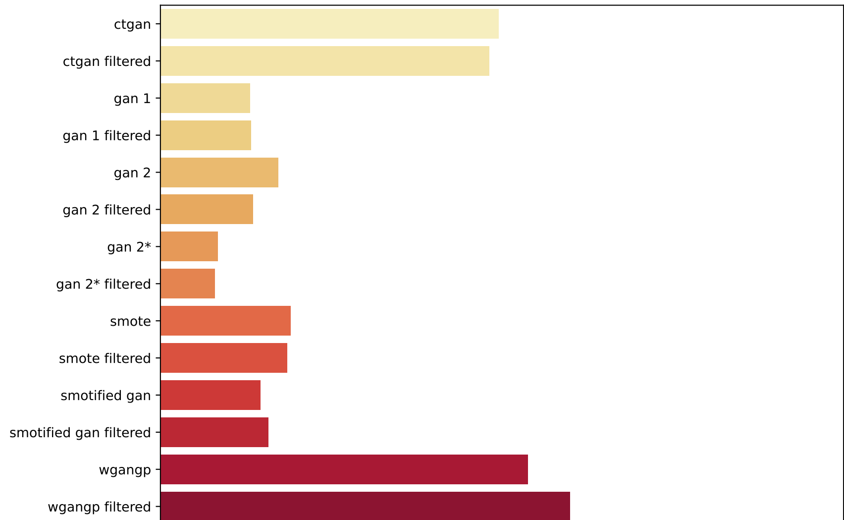
IQR Sonar
