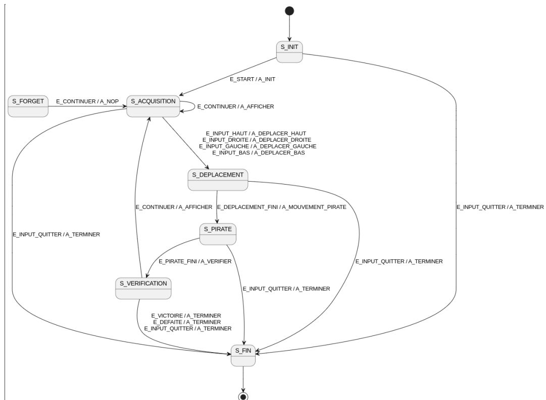
Fig.2 : Diagramme de machine à état
