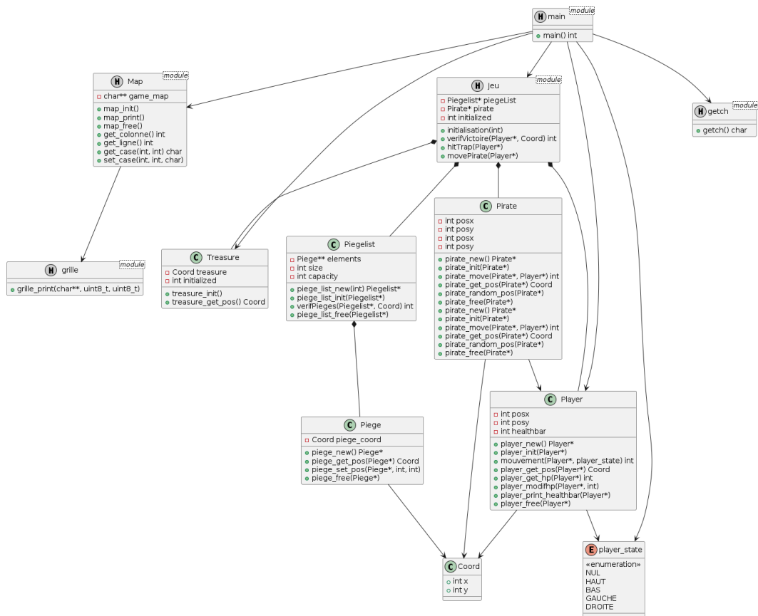
Fig.1 : Diagramme de classe
