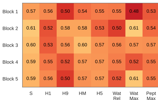
(d) AUC by descriptor: activity cliffs
