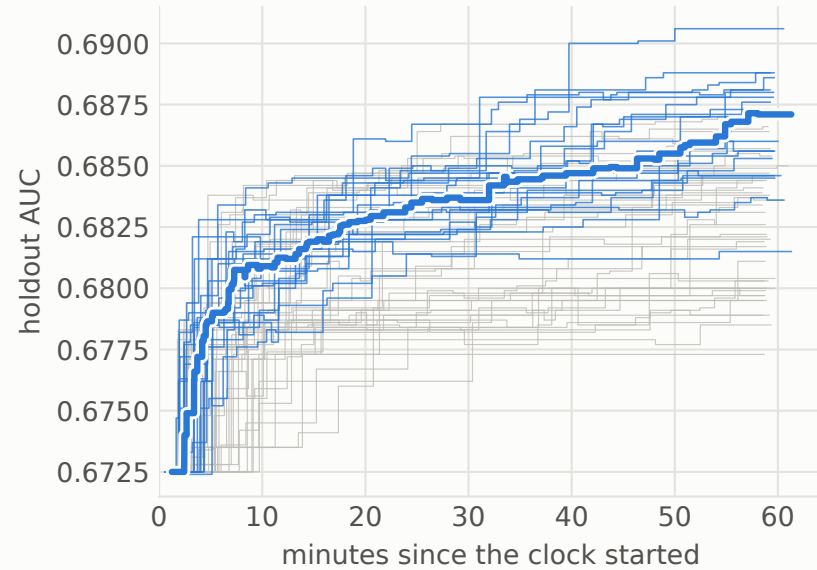
gpt-6-astra
