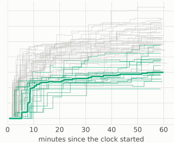
gpt-6-luna
