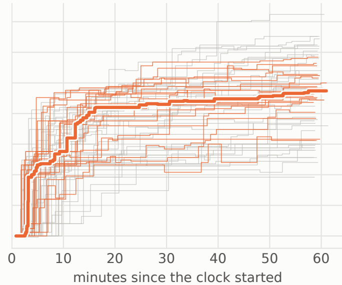
gpt-6-sol
