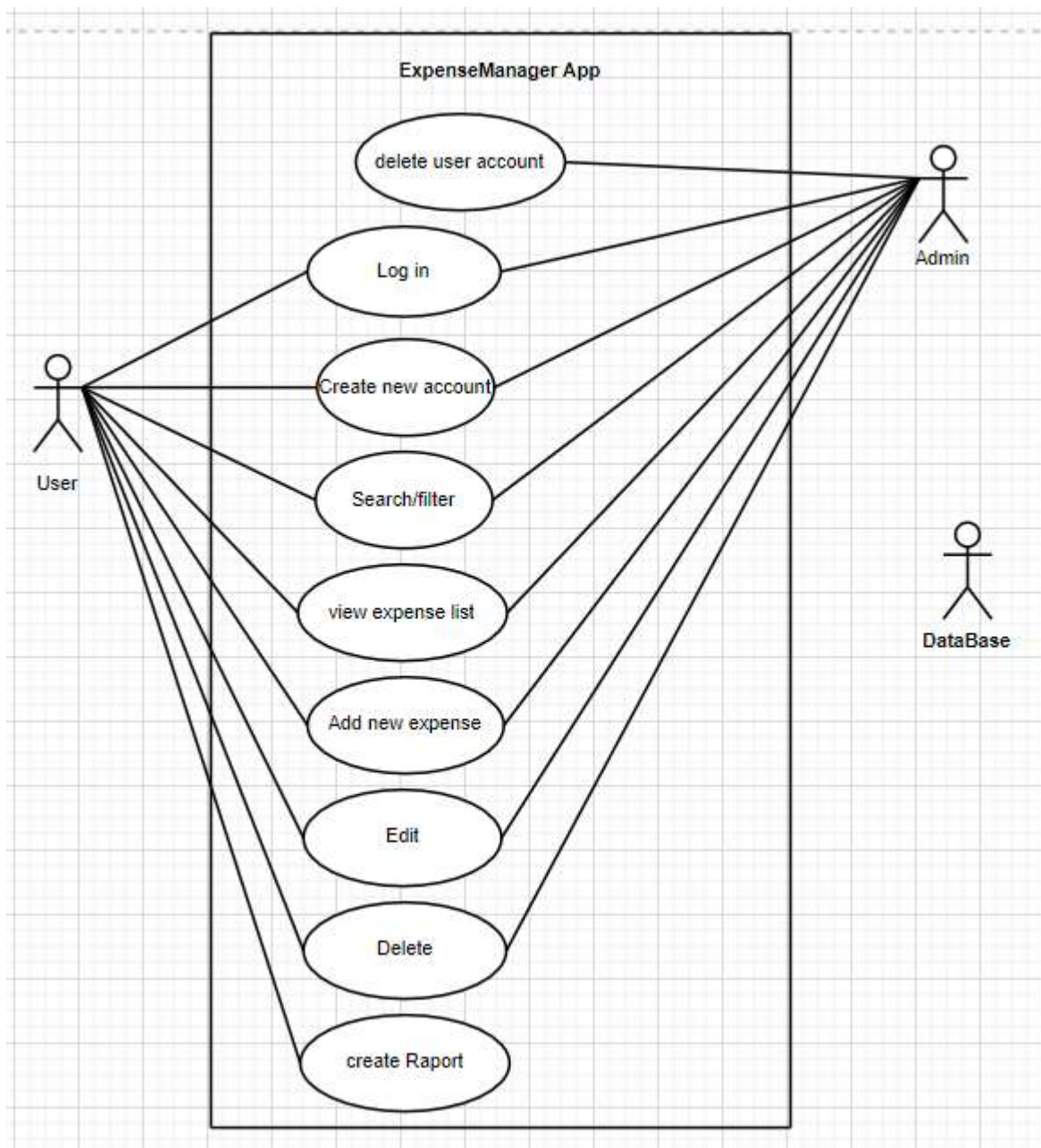
Rysunek 2. Use case diagram.
