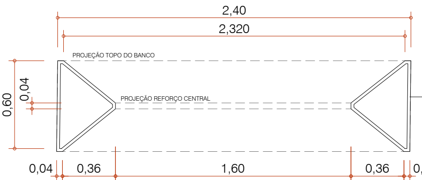
PLANTA BANCO - APOIO ESC 1:25
