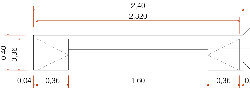
VISTA FRONTAL ESC 1:25
