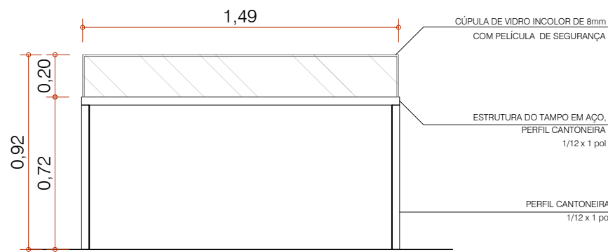
VISTA FRONTAL ESC 1:25
