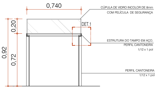
CORTE ESC 1:25
