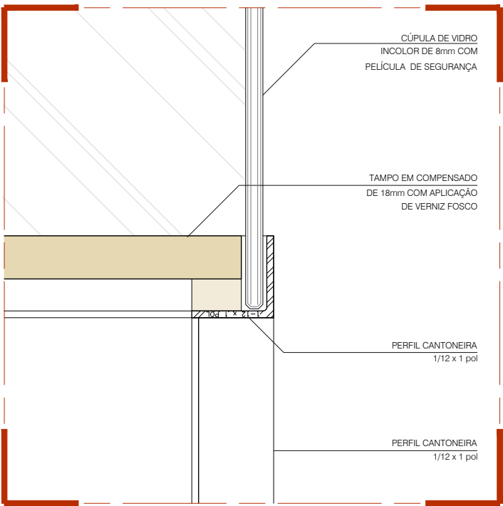
DETALHE 01 ESC 1:2,5
