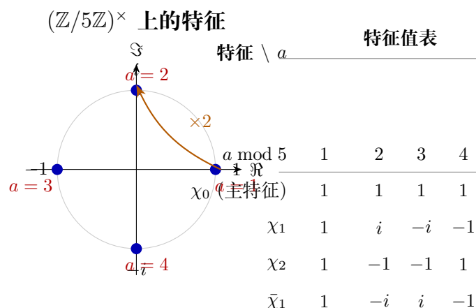
图 2.4: 模 5 的 Dirichlet 特征。$(\mathbb{Z}/5\mathbb{Z})^\times = \{1, 2, 3, 4\}$ 是循环群，生成元 2 (因为 $2^1 = 2, 2^2 = 4, 2^3 = 3, 2^4 = 1 \pmod{5}$)。共有 4 个特征，对应四次单位根 $\{1, i, -1, -i\}$ (左侧单位圆)。 \chi_0 是主特征， \chi_1 是将生成元 2 映到 i 的特征。所有特征延拓到 \mathbb{Z} 上时，令 \chi(n) = 0 若 \gcd(n, 5) > 1 。
