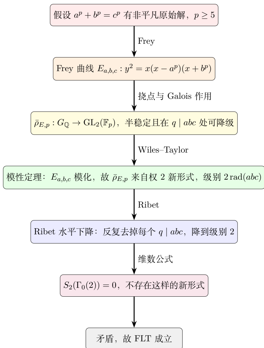
图 9.1: 费马大定理证明中的 Galois 表示路线图：从 Frey 曲线出发，经模性与水平下降，最终落到空的空间 S_2(\Gamma_0(2)) 。
