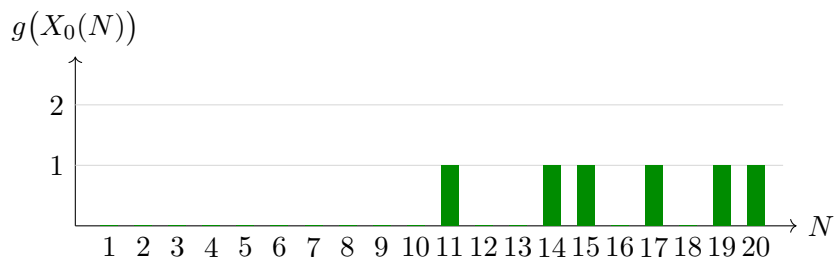
图 5.4: X_0(N) 的亏格在小级别的分布。直到 N = 10 都还是亏格 0; 从 N = 11 开始, 权 2 cusp form 才真正稳定出现。
