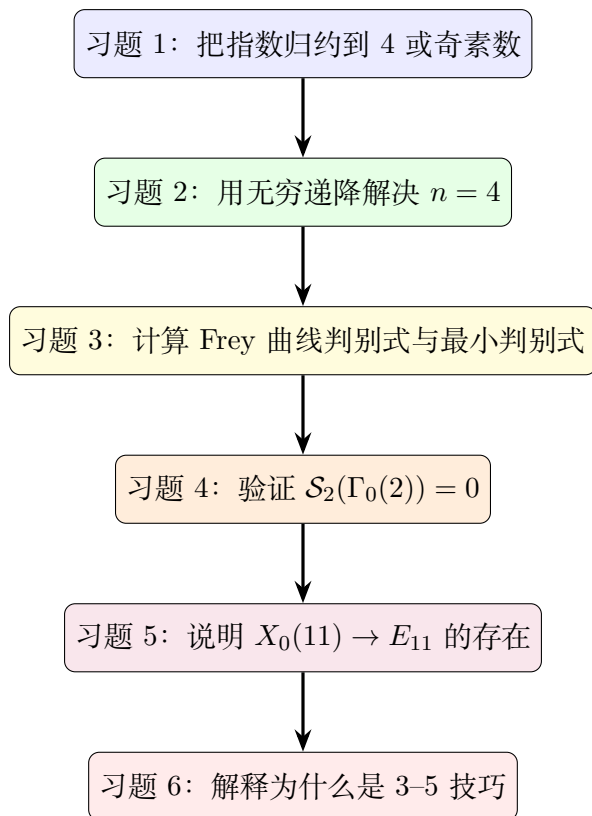
图 10.8: 终章习题的路线图：从指数归约与无穷递降出发，经 Frey 曲线与空空间 S_2(\Gamma_0(2)) ，最后回到 Wiles 证明中最精巧的 3-5 技巧。
