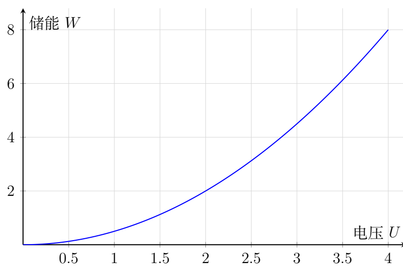
图 9.5: 电容器储能随电压呈抛物线增长
