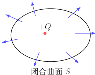
图 8.2: 高斯面与穿出闭合曲面的电场通量
