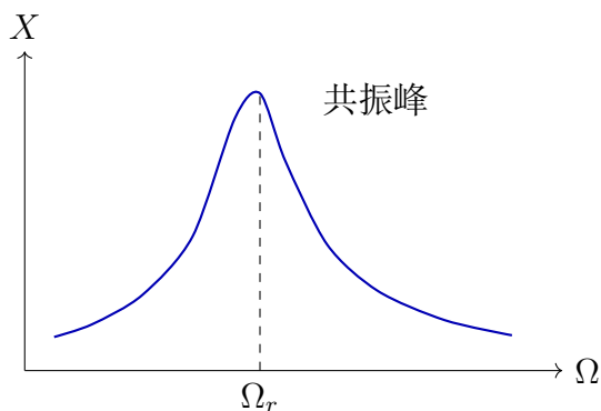
图 7.3: 阻尼受迫振动的振幅—频率曲线示意图
