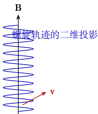
图 11.4: 带电粒子斜射入匀强磁场时的螺旋运动示意
