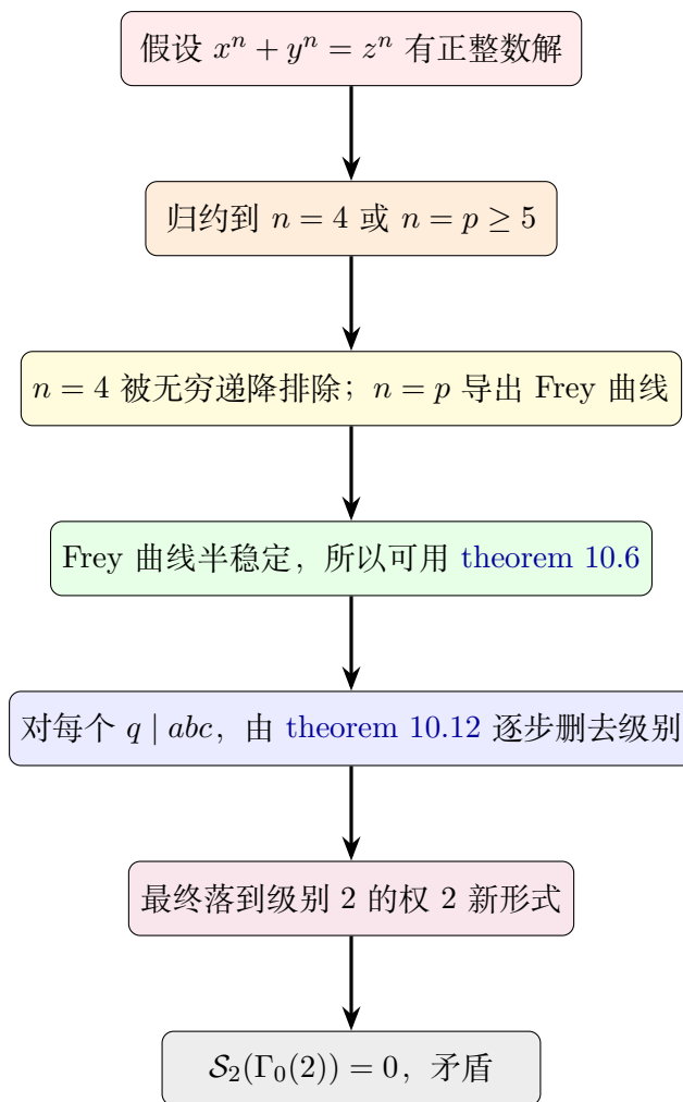
图 10.6: 费马大定理证明的完整链条: 假想解先被归约到奇素数指数, 再经 Frey 曲线、模性与水平下降一路走向空空间。
