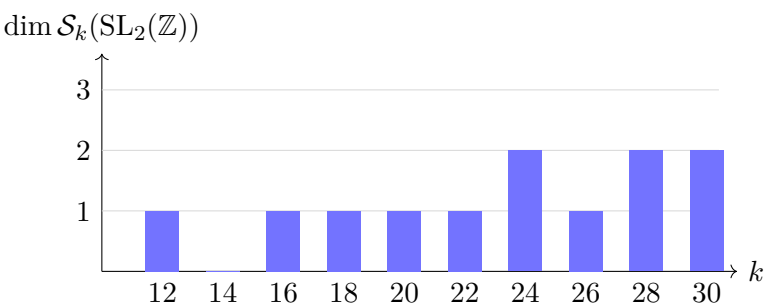
图 5.1: \mathrm{SL}_2(\mathbb{Z}) 上尖点形式空间维数的前几个值。最早出现的非零空间是 \mathcal{S}_{12} = \mathbb{C}\Delta ；之后维数按“每跨过一个 12 就大致增加 1”的节奏增长。
