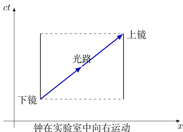
图 14.5: 实验室参考系中运动光钟的折线光路
