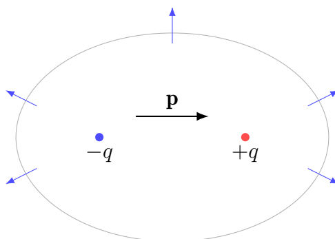
图 8.5: 电偶极子及其远处电场分布示意
