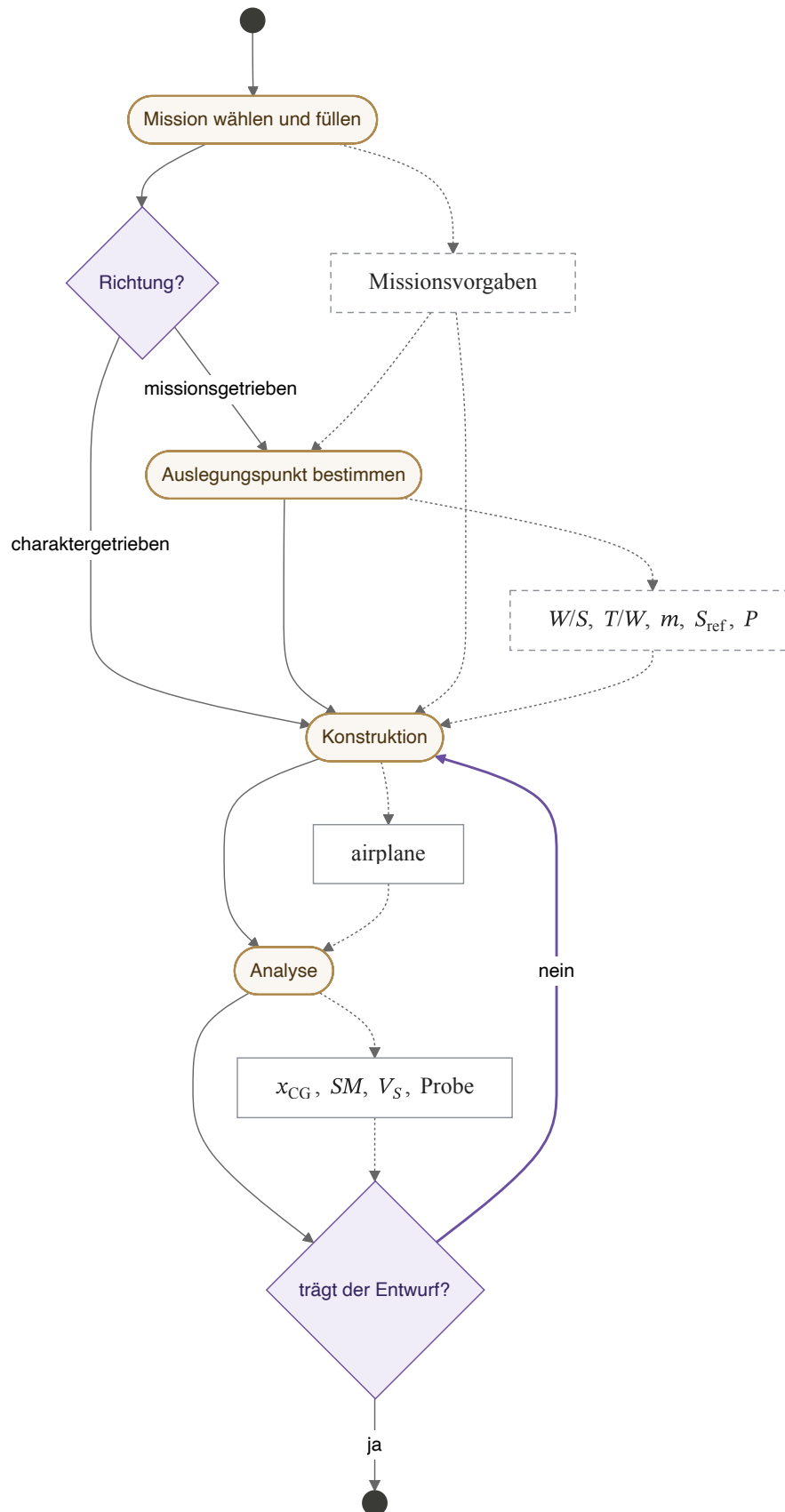
Abbildung 1: Der Ablauf des Anwenders. Rauten sind seine Entscheidungen; der violette Rückweg ist der Entwurfszyklus und hat bewusst keinen rechenbaren Wächter. Gestrichelte Pfeile sind Objektfluss, gestrichelte Kästen Werte, deren Inhalt noch offen ist.
