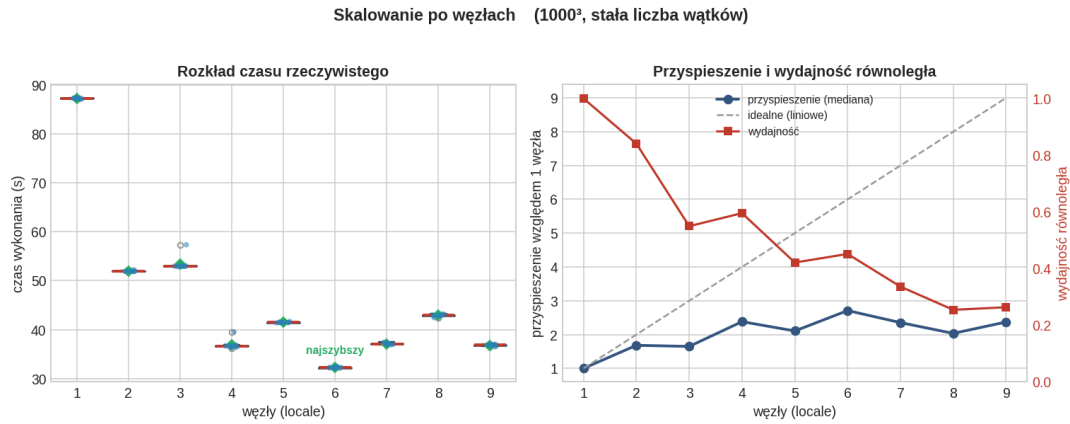
Rysunek 5.2: Skalowanie liczbą węzłów dla dziedziny 1000 3 . Lewy panel: rozkład czasu wykonania w funkcji liczby węzłów. Prawy panel: przyspieszenie na tle przyspieszenia idealnego oraz wydajność E .
