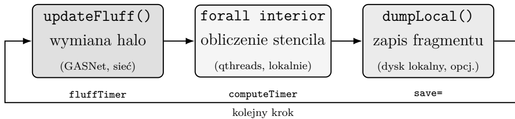
Rysunek 3.2: Potok pojedynczego kroku czasowego programu. Faza komunikacyjna ( updateFluff ) poprzedza lokalne obliczenie stencilu, po którym następuje opcjonalny zapis fragmentu na dysk lokalny. Każda faza mierzona jest osobnym stoperem.
