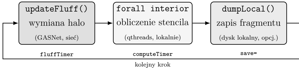
Rysunek 3.2: Potok pojedynczego kroku czasowego programu. Faza komunikacyjna ( updateFluff ) poprzedza lokalne obliczenie stencila, po którym następuje opcjonalny zapis fragmentu na dysk lokalny. Każda faza mierzona jest osobnym stoperem.
