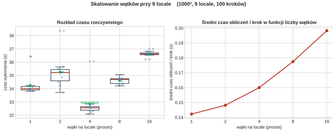
Rysunek 4.4: Skalowanie wątkowe przy dziewięciu węzłach, dziedzina 1000 3 . Lewy panel: rozkład czasu wykonania. Prawy panel: średni czas obliczeń na krok w funkcji liczby wątków, rosnący skutek rywalizacji o zasoby współdzielone.
