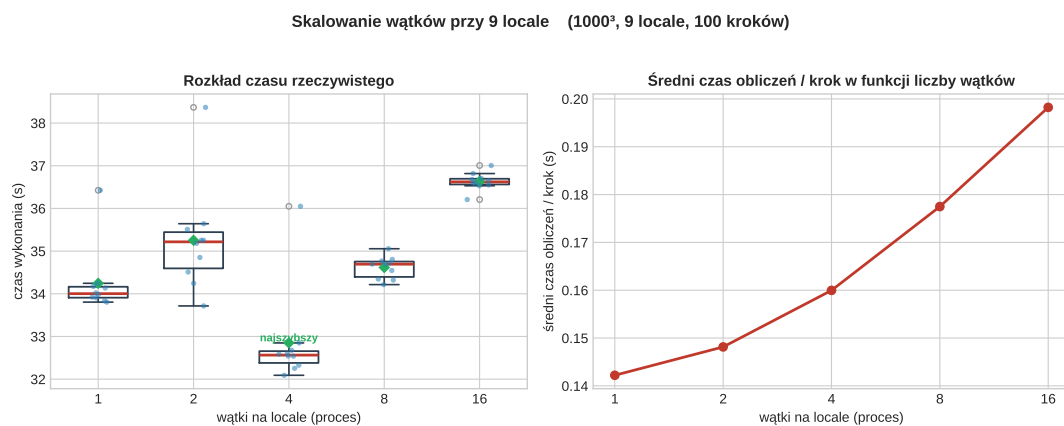
Rysunek 5.4: Skalowanie wątkowe przy dziewięciu węzłach, dziedzina 1000 3 . Lewy panel: rozkład czasu wykonania. Prawy panel: średni czas obliczeń na krok w funkcji liczby wątków, rosnący wskutek rywalizacji o zasoby współdzielone.
