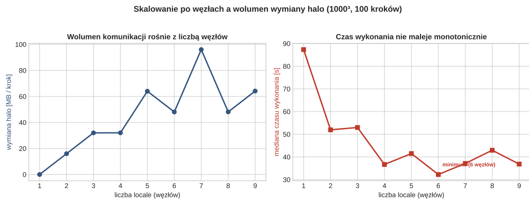
Rysunek 5.3: Objętość warstw brzegowych wymienianych na krok w megabajtach oraz mediana czasu wykonania w funkcji liczby węzłów.
