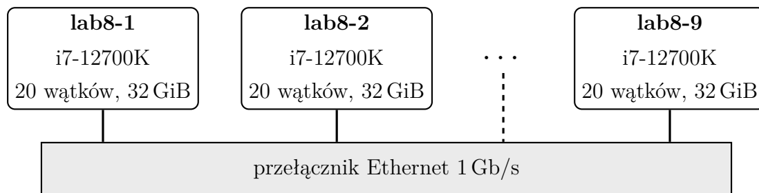
Rysunek 3.1: Topologia jednorodnego, dziewięciowęzłowego klastra Pioneer. Wszystkie identyczne węzły ( Pionier-lab8-1 ... Pionier-lab8-9 ) połączone są jednym przełącznikiem 1 Gb/s, który stanowi współdzielone i zarazem najwęższe łącze komunikacji rozproszonej. Środowisko budowane jest raz na dowolnym węźle, a pliki wykonywalne rozprowadzane na pozostałe.
