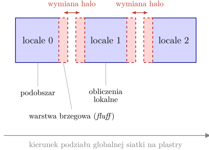
Rysunek 2.3: Dekompozycja dziedziny w postaci plastrów (ang. slab decomposition ) na trzy jednostki ( locale ). Globalna siatka jest cięta wzdłuż jednej osi, którą wskazuje strzałka na dole. Każdy podobszar, zaznaczony na niebiesko, otoczony jest warstwą komórek brzegowych fluff , zaznaczoną na czerwono linią przerywaną, przechowującą kopie krawędzi sąsiadów. Przed każdym krokiem obliczeń warstwy brzegowe są odświeżane w ramach wymiany z najbliższymi sąsiadami.
