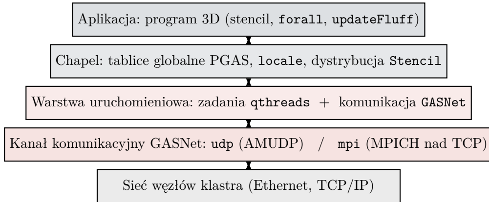
Rysunek 2.4: Warstwowa architektura wykonania. Kod aplikacji operuje na globalnych tablicach PGAS języka Chapel. Ich dostępy zdalne i wymiana warstw brzegowych są realizowane przez warstwę uruchomieniową, w której zadania qthreads wykonują się lokalnie, a komunikacja GASNet zachodzi między węzłami. Warstwa ta korzysta z kolei z wybranego kanału komunikacyjnego odwzorowującego operacje na fizyczną sieć klastra.
