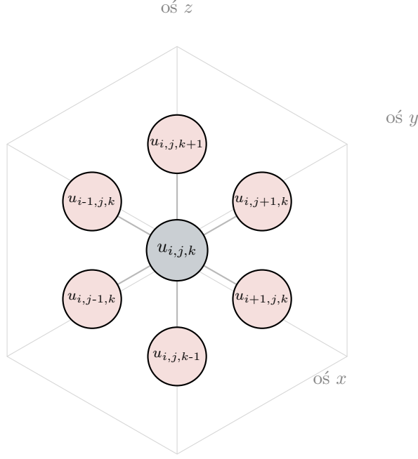
Rysunek 2.2: Siedmiopunktowy stencil trójwymiarowy. Nowa wartość w komórce centralnej u_{i,j,k} , zaznaczonej na niebiesko, jest ważoną kombinacją jej wartości bieżącej oraz sześciu bezpośrednich sąsiadów zaznaczonych na czerwono, wzdłuż osi x , y i z , zgodnie z równaniem (2.5).
