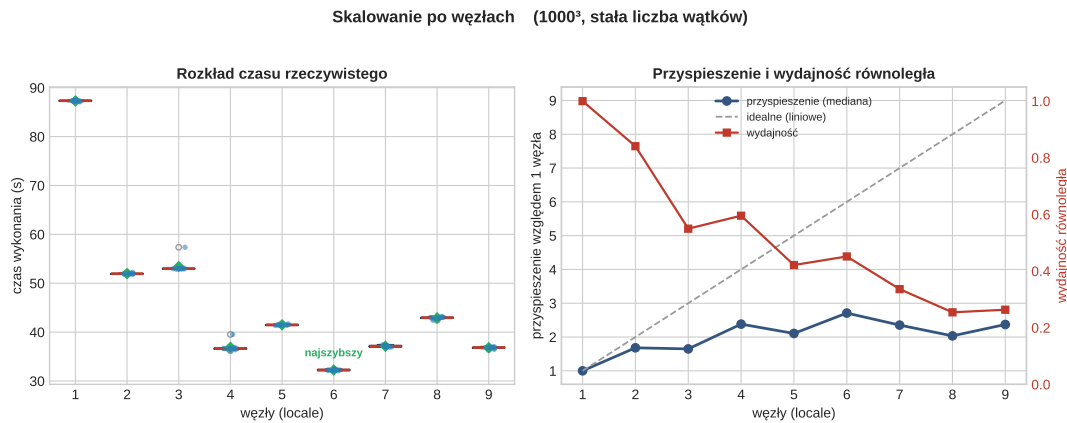
Rysunek 4.2: Skalowanie liczbą węzłów dla dziedziny 1000^3 . Lewy panel: rozkład czasu wykonania w funkcji liczby węzłów. Prawy panel: przyspieszenie na tle przyspieszenia idealnego oraz wydajność E .
