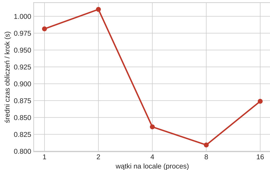
Średni czas obliczeń / krok w funkcji liczby wątków
